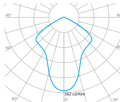
Krzywa rozsyłu światłości oprawy ROLL-M cd/klm — C0 - C180/ C90 - C270
